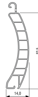
Profil RE 52
